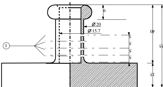
Joon. 3: Õõnes pronksisilinder, ühest otsast suletud; mõõdud mm-tes
